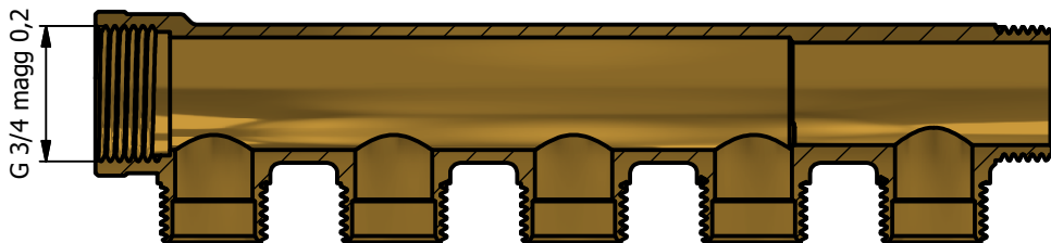
B-B ( 1 : 1.6 )
