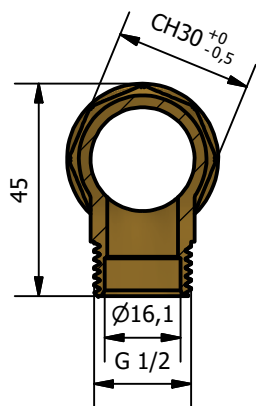
A-A ( 1 : 1.6 )
