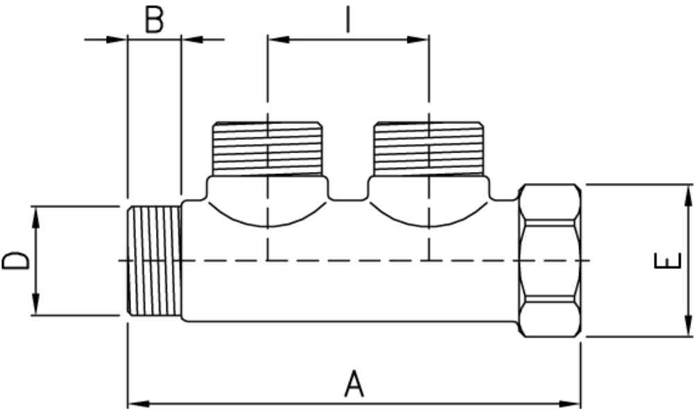
Collettori con derivazione maschio - interasse 36. Manifolds lateral male connection - center distance 36 mm.
