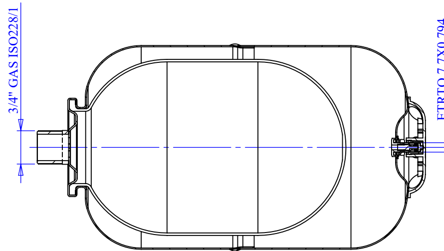
SEZIONE E-E
