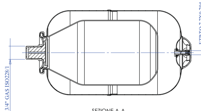
SEZIONE A-A
