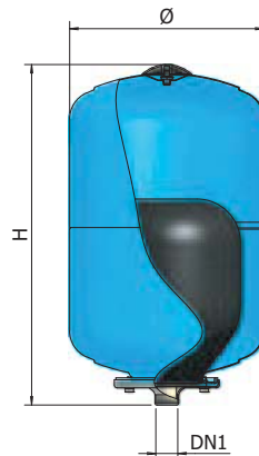
AC 5 - 25; AFV 24
