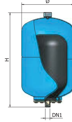
AC 20 PN25
