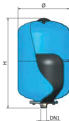
AC 5 - 25; AFV 24
