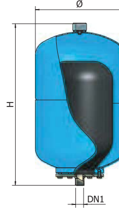
AC 20 PN25
