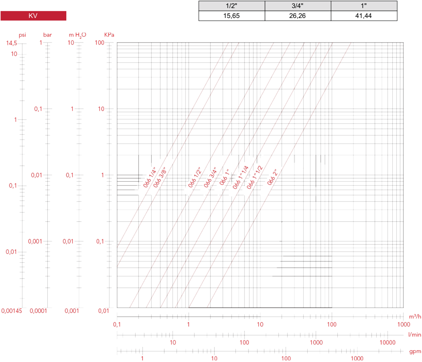
DIAGRAMMA PERDITE DI CARICO (Con acqua)
