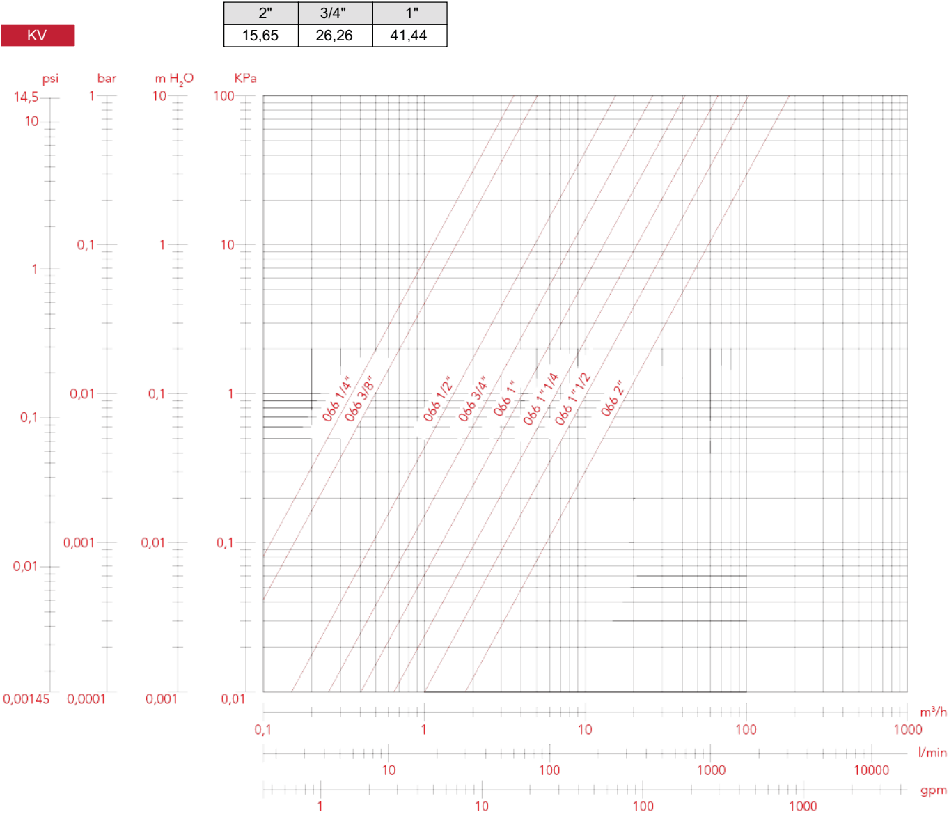
DIAGRAMMA PERDITE DI CARICO (Con acqua) misure da 1/4" a 2"
